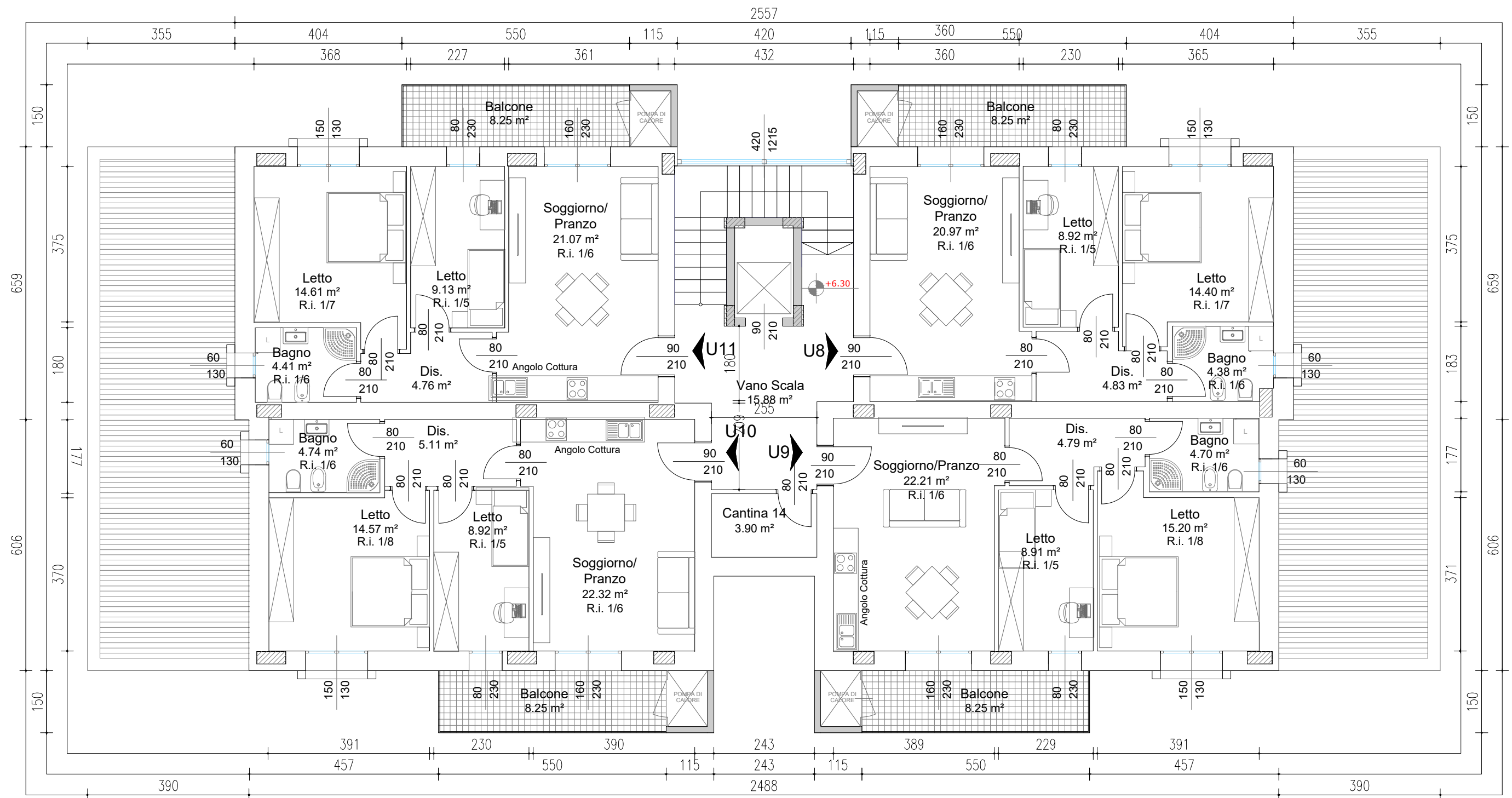
PIANTA PIANO SECONDO Scala 1:100
